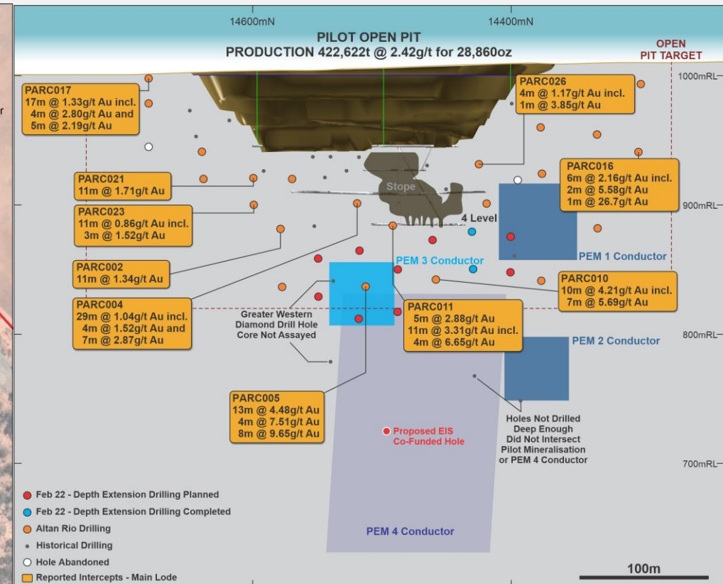
Pilot – Longitudinal Section
